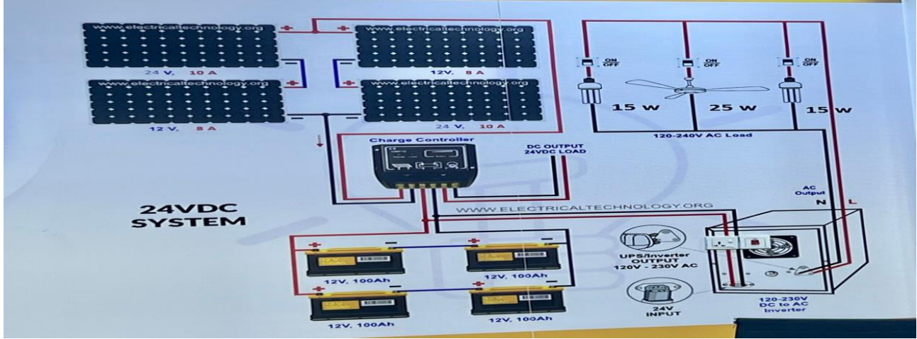
مخطط توضيحي لألية عمل الألواح الشمسية
